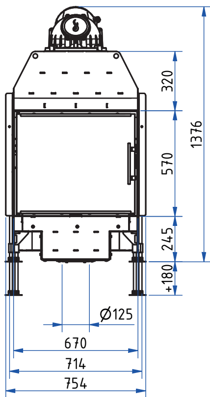
Čelní pohled M 1:20
