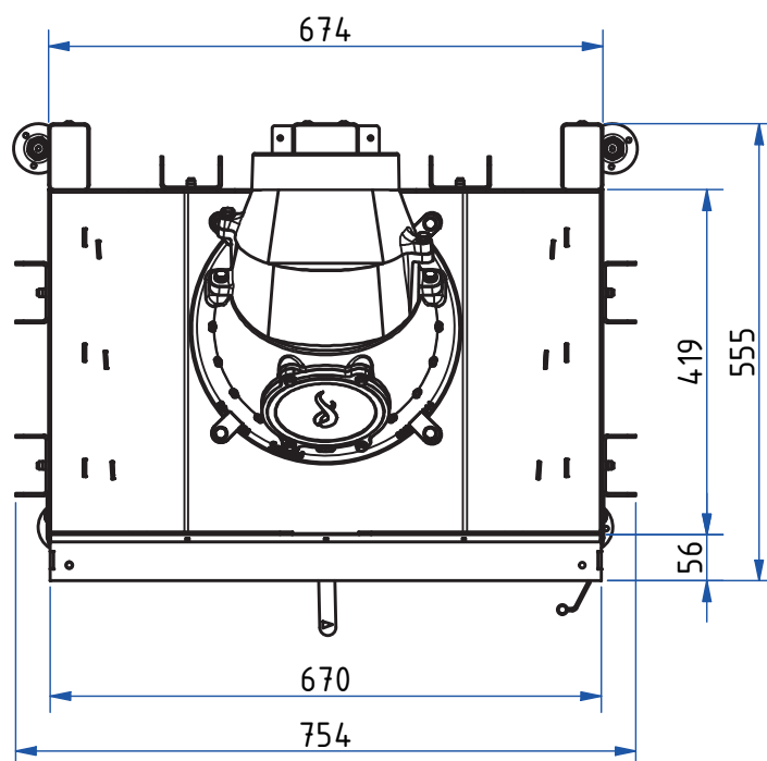
Půdorys M 1:10
