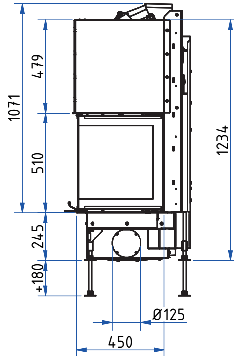
Seitenansicht M 1:20
