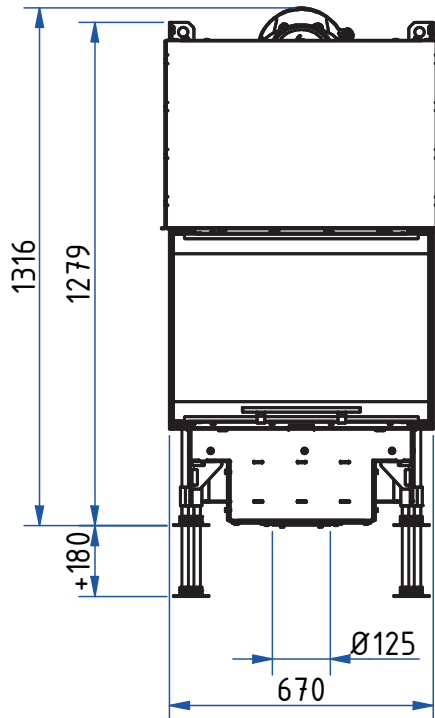
Frontansicht M 1:20
