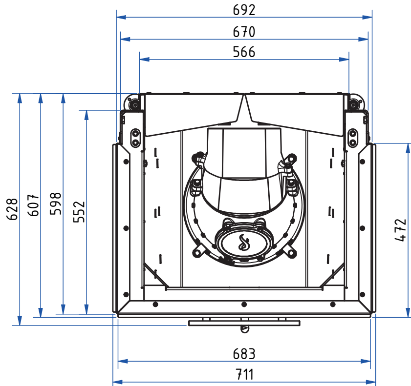
Draufsicht M 1:10
