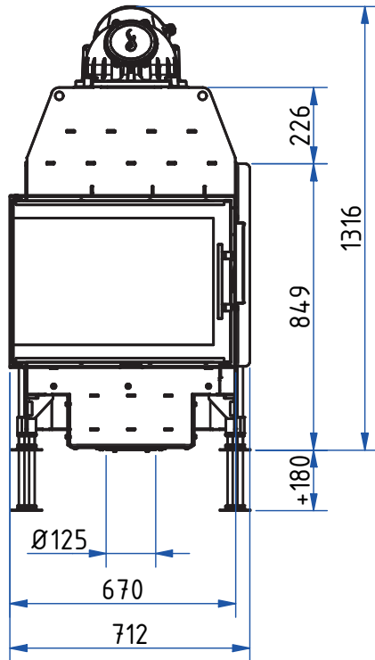
Frontansicht M 1:20
