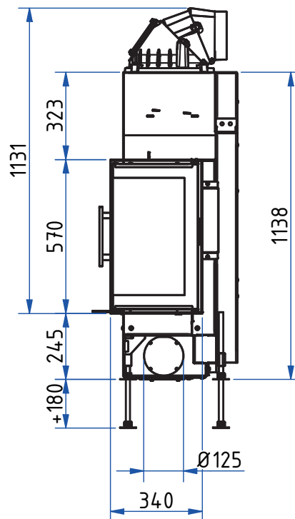
Boční pohled M 1:20
