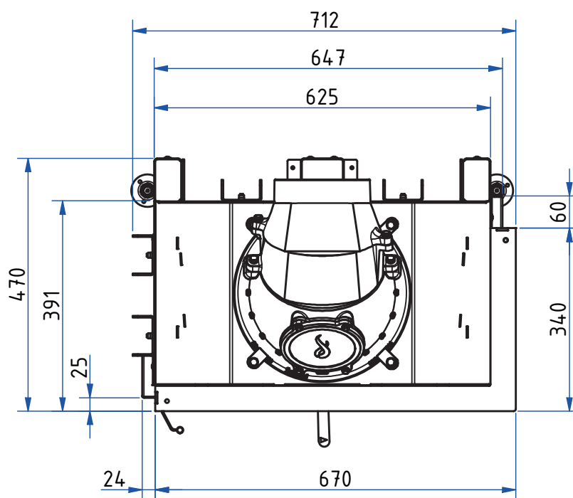
Půdorys M 1:10
