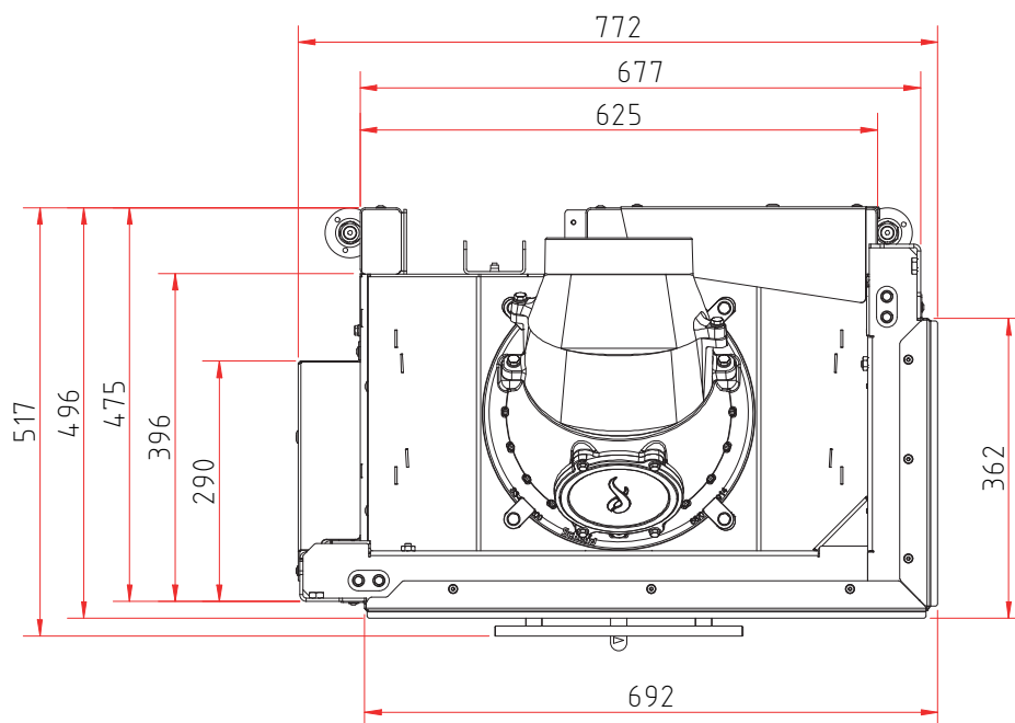
Půdorys M 1:10
