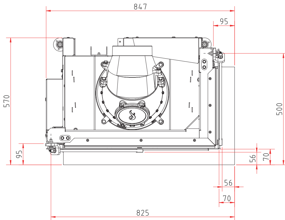
Půdorys M 1:10
