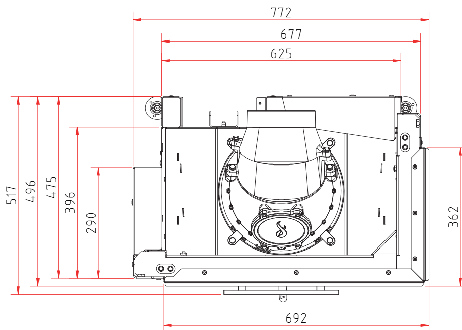
Půdorys M 1:10
