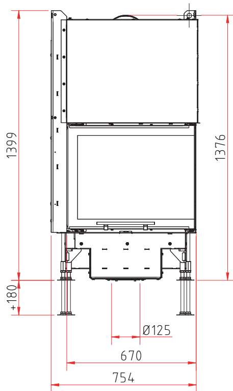
Čelní pohled M 1:20
